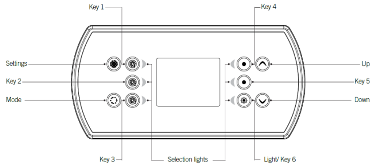
in.k800 keypad layout
